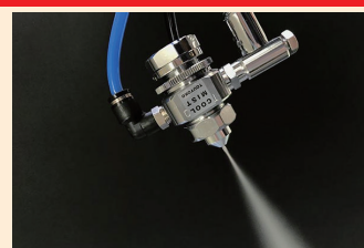
水とエアだけで-8℃ クールミストLine
